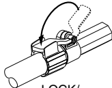
Figure 5 - Comment attacher ensemble le câble de rallonge et le cordon d'alimentation de la scie
